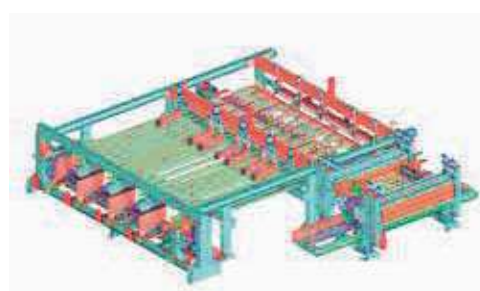
Rifilosquadratrice Modul-SQ / Modul-SQ Trimming-squaring machine
