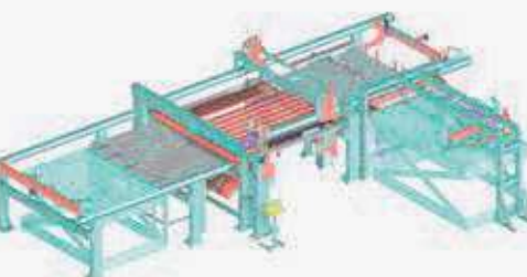
Sezionatrice-rifilatrice per pannelli di compensato e derivati (H 80 mm) Saw blade and trim cut machine for plywood panel (H 80 mm)
